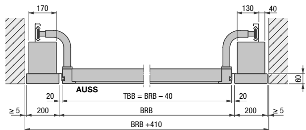
Horizontalschnitt
